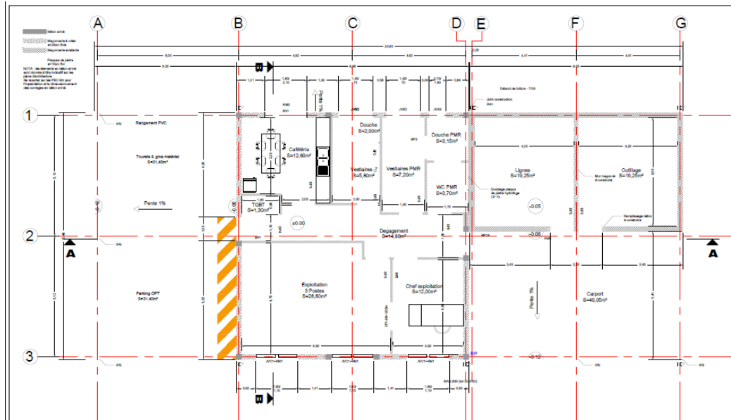
Plan indicatif de l'unité de service de La Roche, Maré
